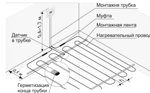
Рисунок 1. Монтаж терморегулятора и теплого пола
